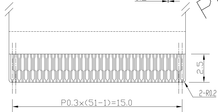
K1 Details (Conductor Side) SCALE=3/1
